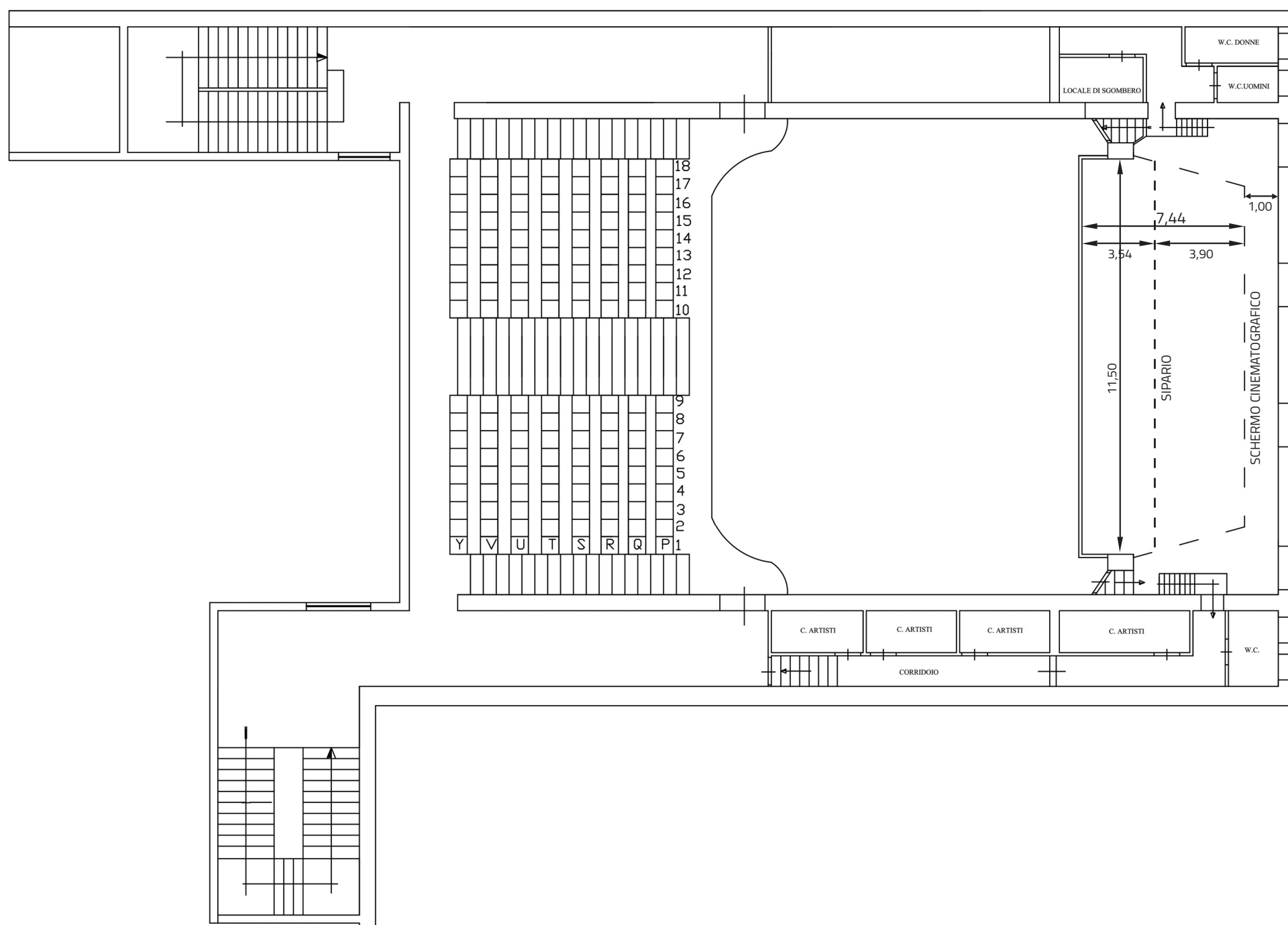
CINE TEATRO GARIBALDI TRIBUNA SCALA 1:100
