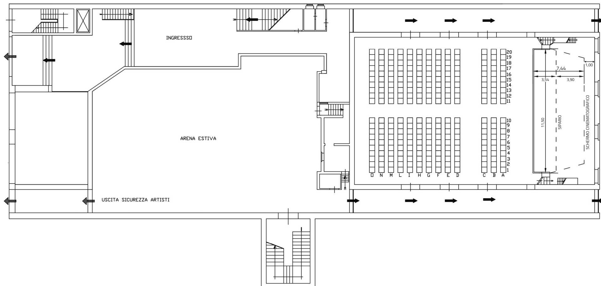
CINE TEATRO GARIBALDI PLATEA SCALA 1:100
